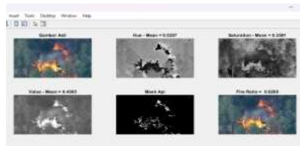
Gambar 2. Hasil Segmentasi
